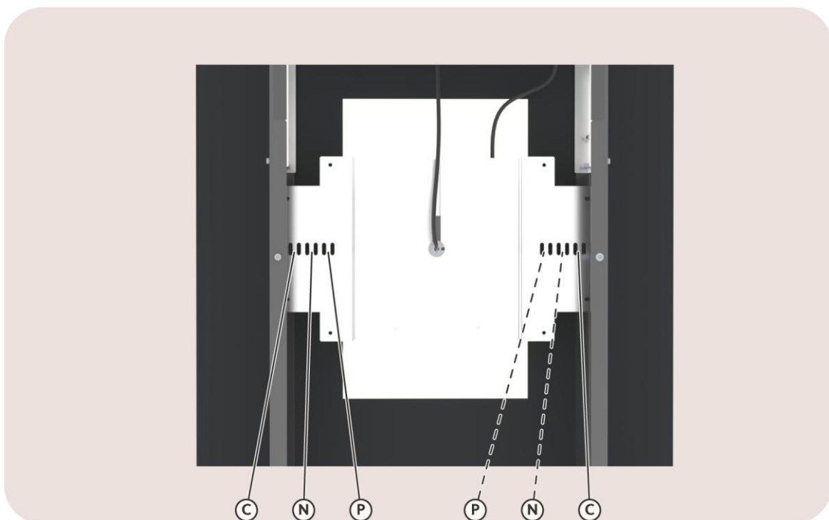
Afbeelding 37: de bevestiging van de voedingskabel (P), de oplaadkabel (C) en de netwerkkabel (N)
