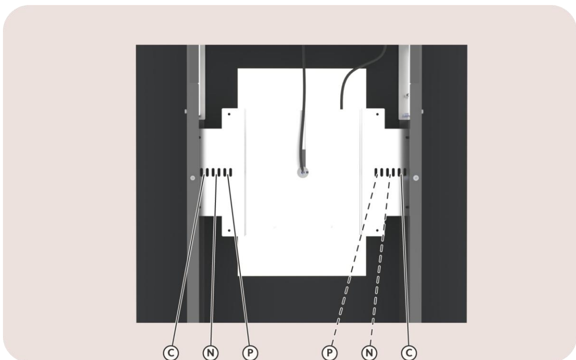
Image 37 : Vue de la fixation du câble d'alimentation (P), du câble de recharge (C) et du câble réseau (N).
