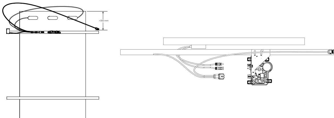
Illustration 3 : Montage vertical
