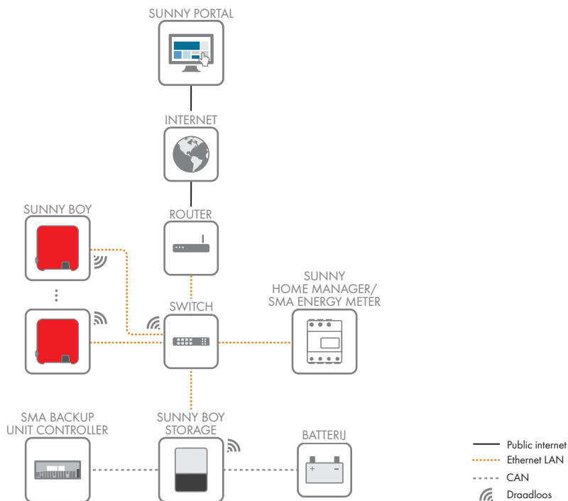
Afbeelding 5: Structuur installatiecommunicatie
