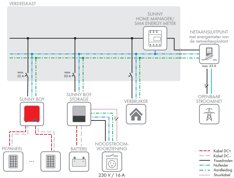
Afbeelding 4: Schakelschema (voorbeeld)
