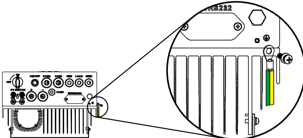
Erdung Anschließen (Kupferdrähte)
